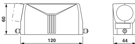
Rysunek wymiarowy
